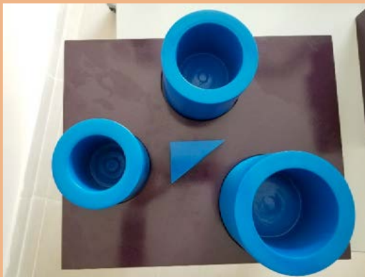
Demstración del Teorema de Pitágoras con cilindros
